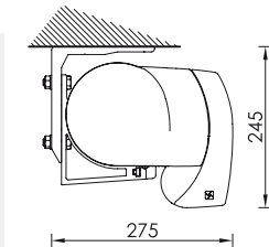
Montaggio a soffitto con terminale a cassettono Ceiling installation with box terminal bar
