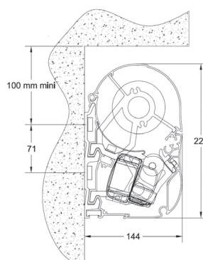
Ecombement de la banne mini
